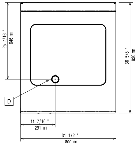
Felülnézet
